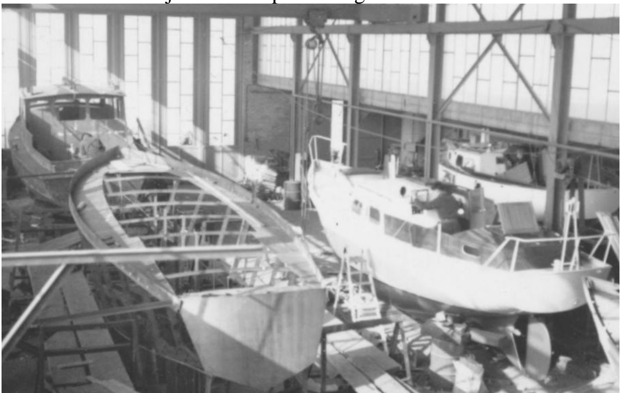
De naar voren geschoven en nu bijna gereed zijnde werkvlet. Daarachter een van de drie in aanbouw zijnde stalen zeiljachten voor Dekker in Aalsmeer , geleverd naar de USA.
